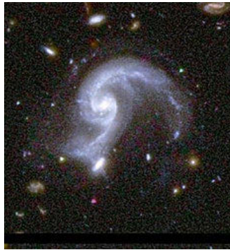
Tres de las 380.000 galaxias catalogadas por Euclid. ESA
